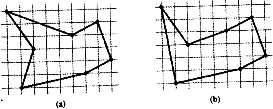
Hình 16.6 Bảy điểm trong mặt phẳng, được nêu trên một khung kẻ ô đơn vị. (a) Chuyến đi khép kín ngắn nhất, có chiều dài 24.88....Chuyến đi này không phải là bitonic. (b) Chuyến đi bitonic ngắn nhất cho cùng tập hợp các điểm. Chiều dài của nó là 25.58....
