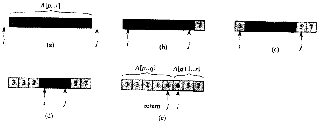
Hình 8.1 Phép toán của PARTITION trên một mảng mẫu. Các thành phần mảng tô bóng sáng đã được đặt vào đúng phân hoạch, và các thành phần tô bóng đậm chưa nằm trong các phân hoạch của chúng. (a) Mảng đầu vào, có các giá trị ban đầu i và j vượt ra khỏi các đầu trái và phải của mảng. Ta phân hoạch quanh x = A[p] = 5 . (b) Các vị trí của i và j tại dòng 9 của lần lặp đầu tiên của vòng lặp while . (c) Kết quả của việc trao đổi các thành phần được i và j trở đến trong dòng 10. (d) Các vị trí của i và j tại dòng 9 của lần lặp thứ hai của vòng lặp while . (e) Các vị trí của i và j tại dòng 9 của lần lặp lại thứ ba và chót của vòng lặp while . Thủ tục kết thúc bởi vì i \geq j , và giá trị q = j được trả về. Các thành phần mảng lên đến và kể cả A[j] sẽ nhỏ hơn hoặc bằng với x = 5 , và các thành phần mảng sau A[j] sẽ lớn hơn hoặc bằng với x = 5 .
