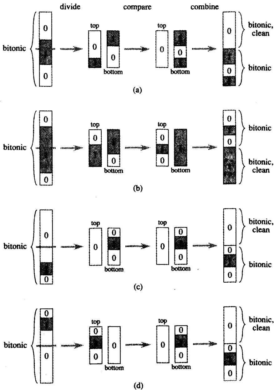
Hình 28.8 Các phép so sánh khả dĩ trong HALF-CLEANER[n]. Dãy nhập liệu được mặc nhận là một dãy bitonic gồm các 0 và 1, và không để mất tính tổng quát, ta mặc nhận rằng nó có dạng 00\dots 011\dots 100\dots 0 . Các dãy con các 0 được tô trắng, và các dãy con các 1 được tô xám. Ta có thể xem n nhập liệu như đang được chia thành hai nửa sao cho với i = 1, 2, \dots, n/2 , các nhập liệu i và i + n/2 được so sánh. (a)-(b) Các trường hợp ở đó xảy ra phép chia trong dãy con giữa của các 1. (c)-(d) Các trường hợp ở đó xảy ra phép chia trong một dãy con các 0. Với tất cả các trường hợp, mọi thành phần trong nửa trên ít nhất nhỏ bằng mọi thành phần trong nửa dưới, cả hai nửa đều là bitonic, và ít nhất một nửa là sạch.
