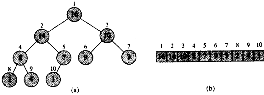
Hình 7.1 Một đống được xem là (a) một cây nhị phân và (b) một mảng. Con số bên trong vòng tròn tại mỗi nút trong cây là giá trị lưu trữ tại nút đó. Con số cạnh một nút là chỉ số tương ứng trong mảng.
