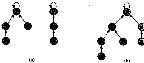
Hình 22.4 Một rừng tập hợp rời. (a) Hai cây biểu thị hai tập hợp của Hình 22.2. Cây bên trái biểu thị cho tập hợp \{b, c, e, h\} , với c làm đại biểu, và cây bên phải biểu thị cho tập hợp \{d, f, g\} , với f làm đại biểu. (b) Kết quả của UNION( e, g ).
