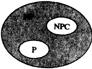
Hình 36.5 Cách thức mà hầu hết các nhà khoa học máy tính lý thuyết xem các mối quan hệ giữa P, NP, và NPC. Cả P lẫn NPC được chứa hoàn toàn trong NP, và P \cap \text{NPC} = \emptyset .
