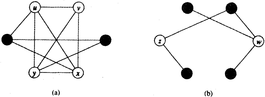
Hình 36.13 Rút gọn CLIQUE thành VERTEX-COVER-(a) Một đồ thị không hướng G = (V, E) có bộ V' = \{u, v, x, y\} . (b) Đồ thị \bar{G} được tạo bằng thuật toán rút gọn có vỏ phủ đỉnh V - V' = \{w, z\} .
