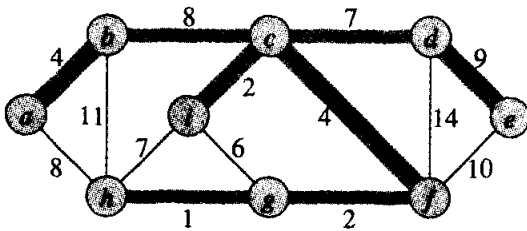
Hình 24.1 Một cây tủa nhánh cực tiểu cho một đồ thị liên thông. Các trọng số trên các cạnh được nêu, và các cạnh trong một cây tủa nhánh cực tiểu được tô bóng. Tổng trọng số của cây được nêu là 37. Cây không phải là duy nhất: việc gỡ bỏ cạnh (b, c) và thay nó bằng cạnh (a, h) sẽ cho ra một cây tủa nhánh khác có trọng số 37.
