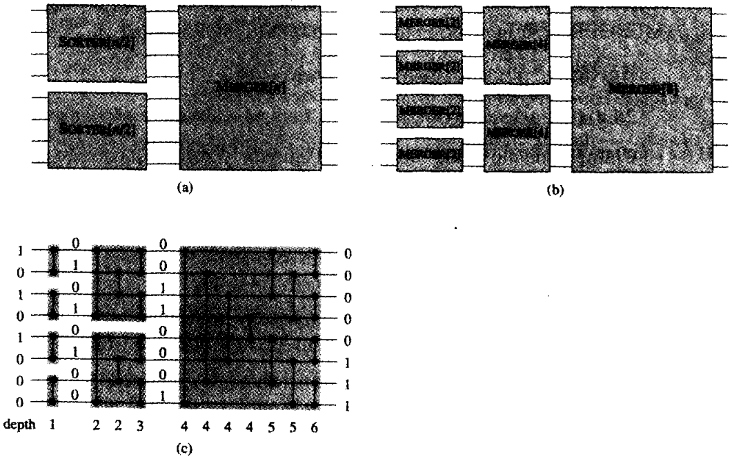
Hình 28.12 Mạng sắp xếp SORTER[n] được kiến tạo bằng cách tổ hợp đệ quy các mạng trộn. (a) Phân kiến tạo đệ quy. (b) Trái rộng phép đệ quy. (c) Thay các hộp MERGER bằng các mạng trộn thực tế. Độ sâu của mỗi bộ so sánh được nêu ra, và các giá trị zero-một mẫu được nêu trên các dây dẫn.
