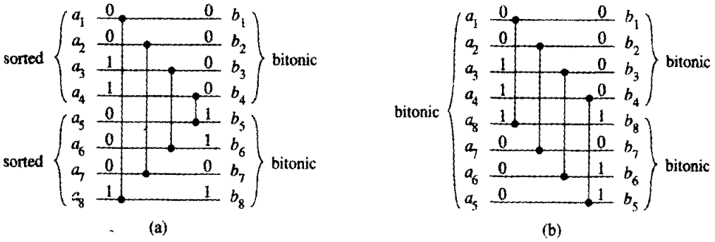
Hình 28.10 So sánh giai đoạn đầu của MERGER[ n ] và HALF-CLEANER[ n ], với n = 8 . (a) Giai đoạn đầu của MERGER[ n ] biến đổi hai dãy nhập liệu monotonic \langle a_1, a_2, \dots, a_{n/2} \rangle và \langle a_{n/2+1}, a_{n/2+2}, \dots, a_n \rangle thành hai dãy bitonic \langle b_1, b_2, \dots, b_{n/2} \rangle và \langle b_{n/2+1}, b_{n/2+2}, \dots, b_n \rangle . (b) Phép toán tương đương cho HALF-CLEANER[ n ]. Dãy nhập liệu bitonic \langle a_1, a_2, \dots, a_{n/2-1}, a_{n/2}, a_n, a_{n-1}, \dots, a_{n/2+2}, a_{n/2+1} \rangle được biến đổi thành hai dãy bitonic \langle b_1, b_2, \dots, b_{n/2} \rangle và \langle b_n, b_{n-1}, \dots, b_{n/2+1} \rangle .
