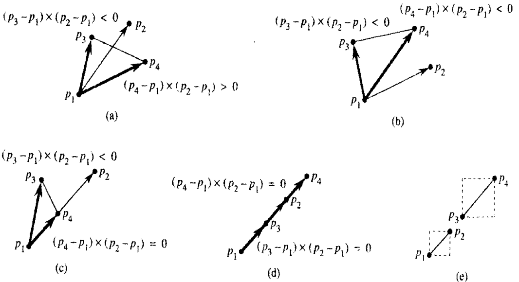
Hình 35.3 Xác định đoạn thẳng \overline{p_1 p_2} cưỡi đường thẳng chứa đoạn thẳng p_3 p_4 . (a) Nếu nó cưỡi, thì các dấu của các tích vectơ (p_3 - p_1) \times (p_2 - p_1) và (p_4 - p_1) \times (p_2 - p_1) khác nhau. (b) Nếu nó không cưỡi, thì các dấu của các tích vectơ giống nhau. (c)-(d) Các trường hợp cận ở đó ít nhất một trong các tích vectơ là zero và đoạn thẳng cưỡi. (e) Một trường hợp cận ở đó các đoạn thẳng là cộng tuyến nhưng không giao nhau. Cả hai tích vectơ là zero, nhưng chúng sẽ không được thuật toán chúng ta tính toán bởi các đoạn thẳng không thể tiến hành đợt kiểm tra phép loại nhanh—các hộp định cận của chúng không giao nhau.
