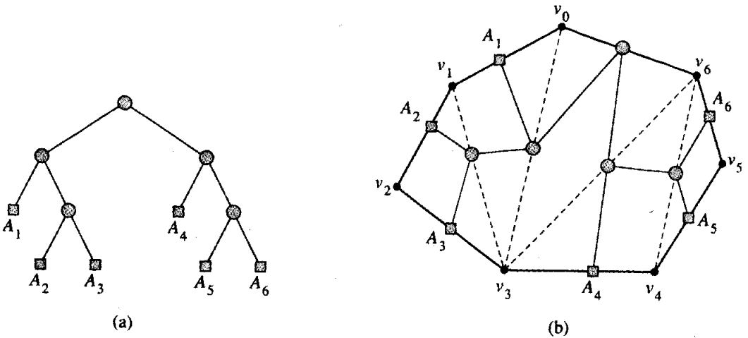
Hình 16.5 Các cây phân ngữ. (a) Cây phân ngữ của tích đã ngoặc đơn ((A_1, (A_2, A_3))(A_4, (A_5, A_6))) và của phép tam giác phân của đa giác có 7 cạnh trong Hình 16.4(a). (b) Phép tam giác phân của đa giác có cây phân ngữ được phủ chồng. Mỗi ma trận A_i tương ứng với cạnh \overline{v_{i-1} v_i} với i = 1, 2, \dots, 6 .
