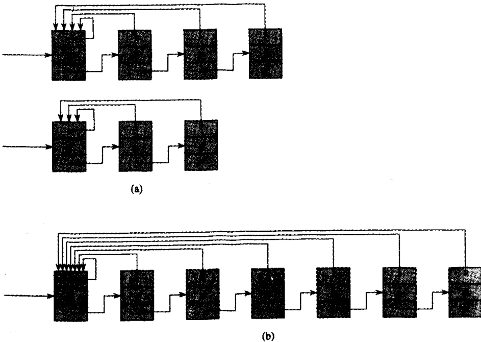
Hình 22.2 (a) Các kiểu biểu diễn danh sách nối kết của hai tập hợp. Một chứa các đối tượng b, c, e, và h, có c làm đại biểu, và một chứa các đối tượng d, f, và g, có f làm đại biểu. Mỗi đối tượng trên danh sách chứa một phần tử tập hợp, một biến trỏ đến đối tượng kế tiếp trên danh sách, và một biến trỏ quay về đối tượng đầu tiên trên danh sách, là đại biểu. (b) Kết quả của UNION(e, g). Đại biểu của tập hợp kết quả là f.
