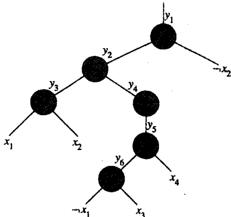
Hình 36.9 Cây tương ứng với công thức
